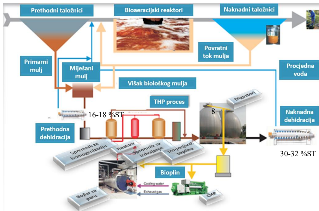
Slika 2. Tehnološka shema linije vode i linije mulja s THP procesom ispred anaerobne digestije ( https://stancelglobal.com/stancelenviro/cambi-thermal-hydrolysis-3/12 )
