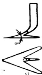
Slika 5. Prikaz tipa motičice - pačje (guščje) nožice (Izvor slike: Strojevi za obradu tla u višegodišnjim nasadima.pptx)
