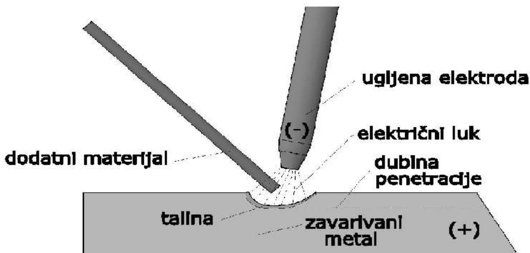
slika 9. Elektrolučno zavarivanje (autor: Mmare)
