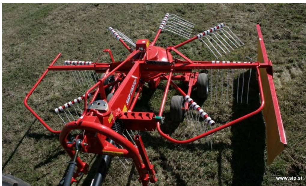
Slika 9. Rotacijske grablje SIP STAR 300/8 ALP (link 5.)
