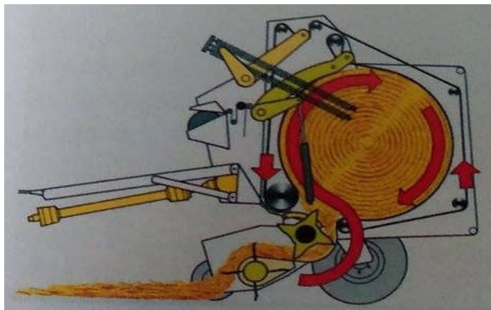
Slika 10. Shema rada prese marke Claas
