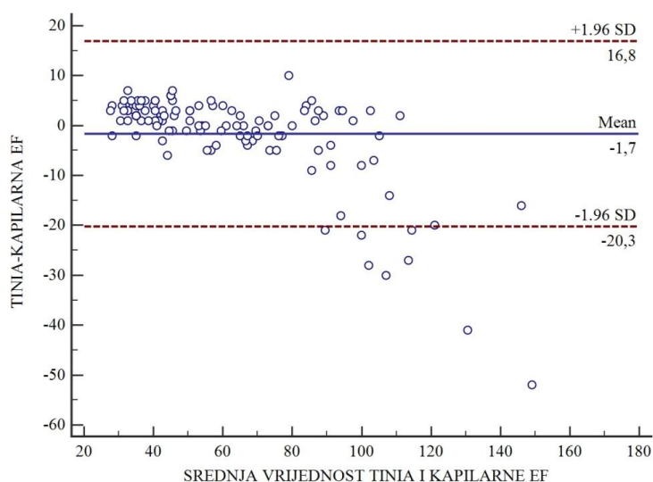
Slika 6: Bland-Altman grafikon
