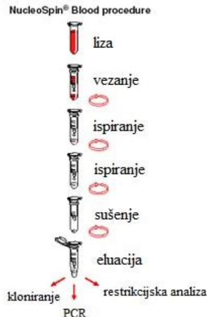
Slika 3. NucleoSpin® Blood mini spin kolona – shema postupka (prilagođeno prema priručniku NucleoSpin® Blood (29))
