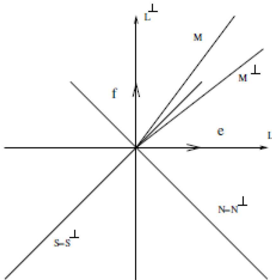
Slika 2.3. Četiri primjera ortogonalnih komplementata u ravнини \mathbb{R}^{1,1} .
