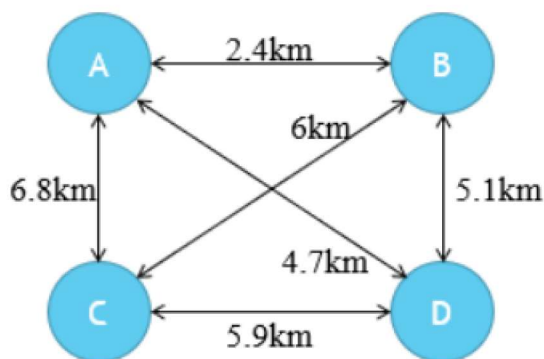
Slika 3.1: Zadani vrhovi i bridovi.
