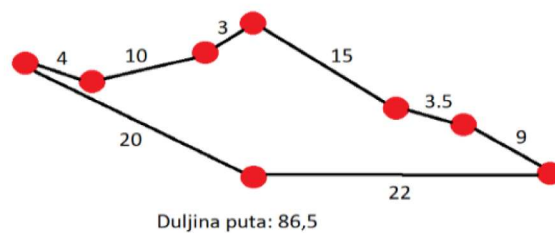
Slika 4.1: Primjer rada 2-opt algoritma
