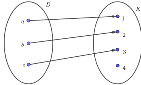
(b) Injekcija, ali nije surjekcija
