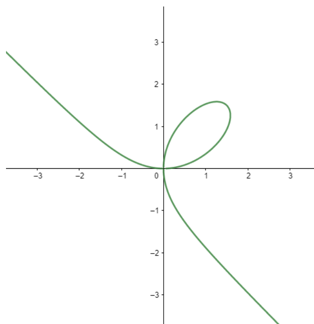
(d) Descartesov list
