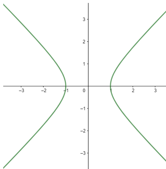
(b) Jednostrana hiperbola
