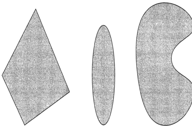
Slika 1: Primjer dva konveksna skupa (s lijeva na desno) i jednog skupa koji nije konveksan
