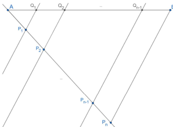
Slika 13: x = \frac{a}{n}
