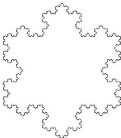
Slika 5.6: Kochova pahulja
