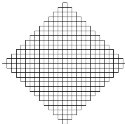
Slika 2.2: Peanova krivulja
