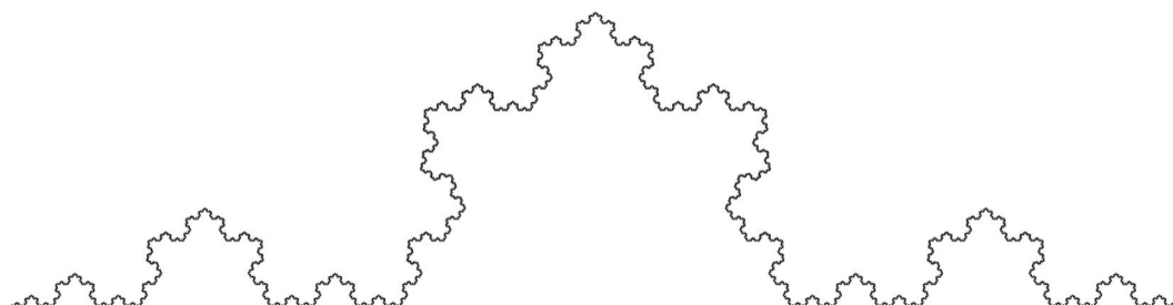
Slika 5.7: Kochova krivulja
