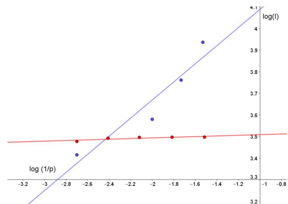
Slika 6.1: log/log graf za obalu i kružnicu
