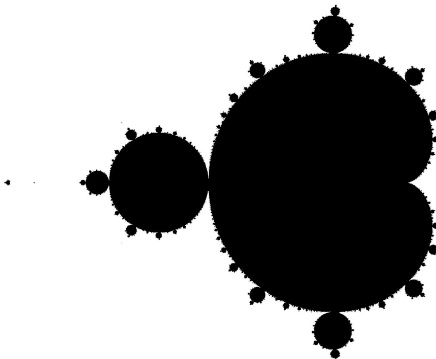
Slika 5.16: Mandelbrotov skup
