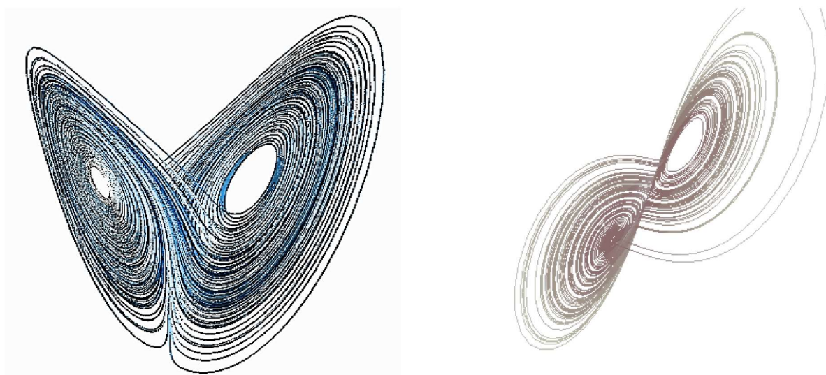
Slika 5.24: Lorenzovi atraktori
