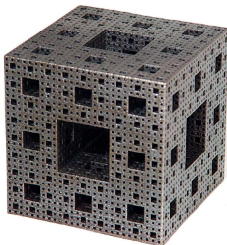
Slika 5.5: Mengerova spužva
