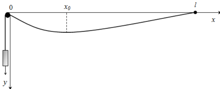
Slika 13: Žica na koju je vezana dodatna žica
