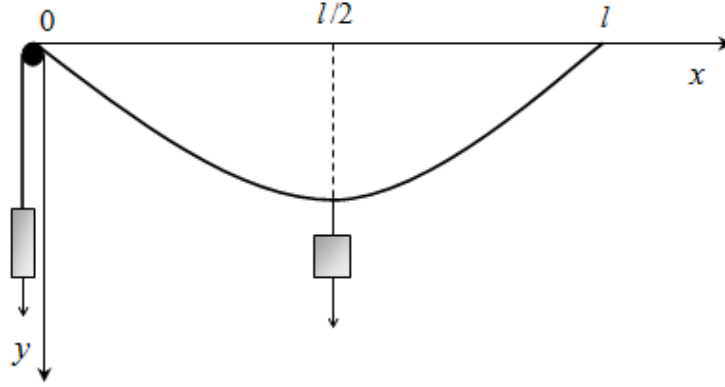
Slika 15: Žica dodatno opterećena utegom mase M_1 u sredini
