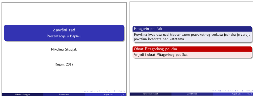
Slika 4.4: Tema Madrid
