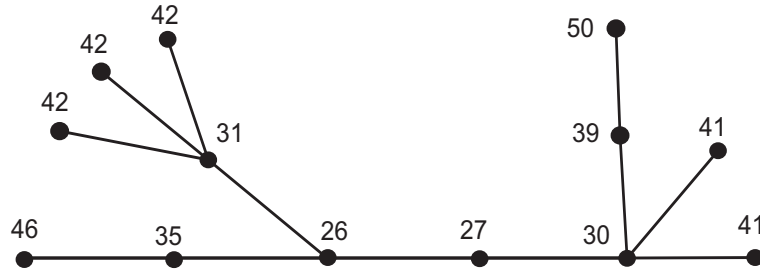
Slika 9: Stablo u kojemu je svakom vrhu v pridružen broj D_T(v) .
