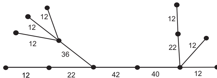
Slika 6: Stablo iz Primjera 2.15.
