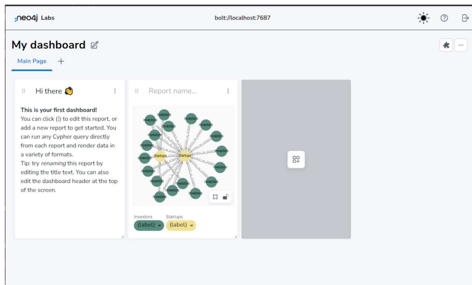
Slika 3.3: Neodash
