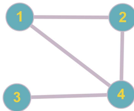
Slika 5.1: Neusmjereni graf
