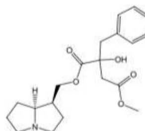
isoretronecanol (4)
