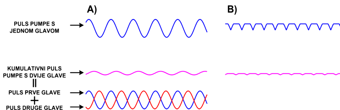
Slika 6. Oblik pulsova uz korištenje pumpi s jednom i dvije glave: A) bez prigušivača i B) s prigušivačem [28].
