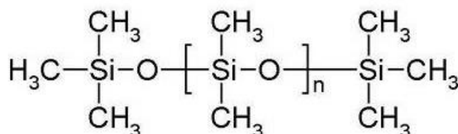
Slika 10. Linearni polidimetilsiloksani
