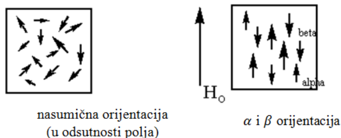
Slika 22. Orijentacije spinova u odsutnosti i prisutnosti polja
