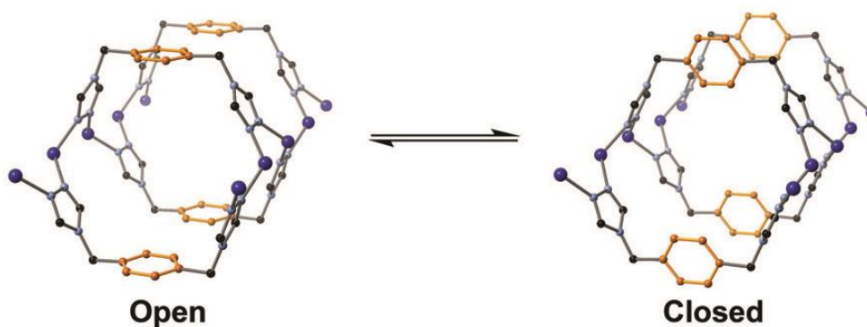
Slika 5. Prikaz dviju različitih vrsta transformacija u MOF-ovima. Rotacijom benzenskog prstena omogućava se prilagođavanje uvjeta/okoline za nadolazeću molekulu gosta [18].
