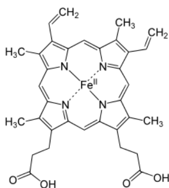
Slika 1. Prikaz kemijske formule hema [10]
