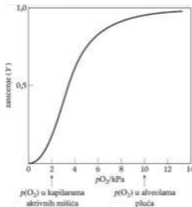
Slika 3. Krivulja vezanja kisika na hemoglobin [7]
