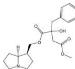
isoretronecanol (4)
