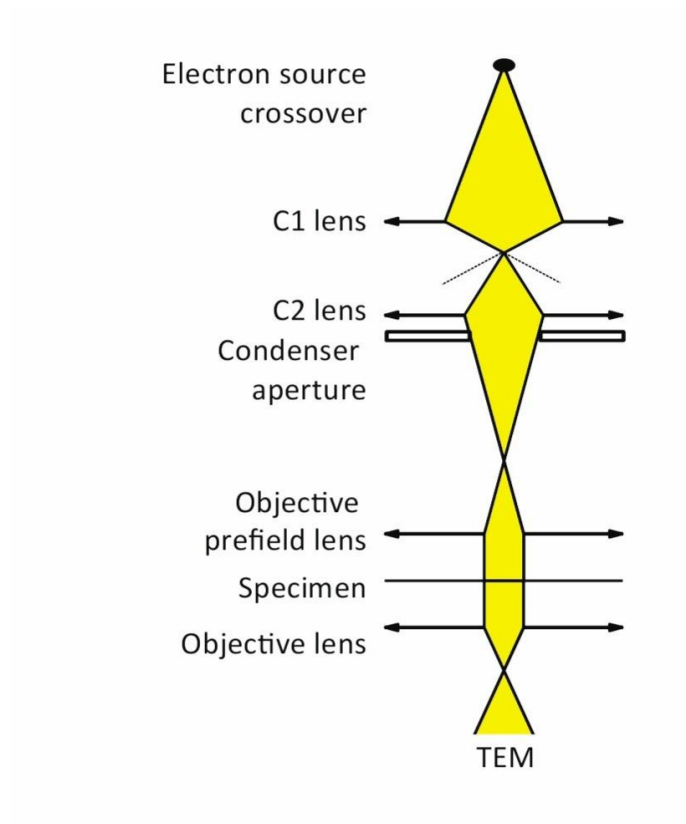
Slika 9. Shema dijelova uređaja za transmisijsku elektronsku mikroskopiju [40].
