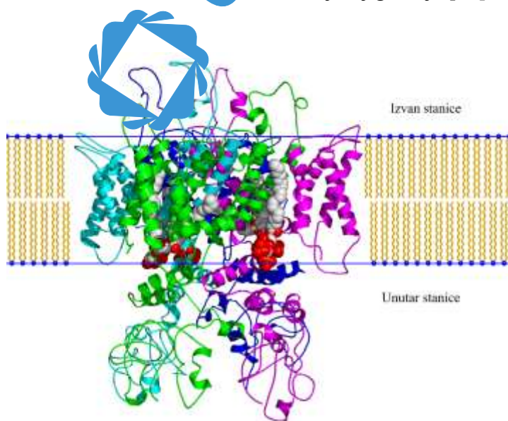
Slika 12. TRPV1 receptor [62].
