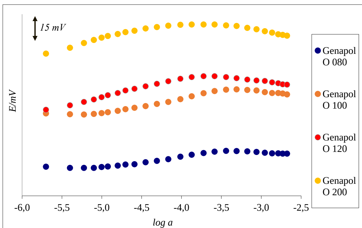
Slika 11. Krivulje odziva DMI-TPB senzora na pseudokationske komplekse Genapola O i \text{Ba}^{2+} pri koncentraciji 0,005M
