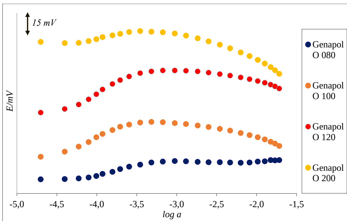
Slika 10. Krivulje odziva DMI-TPB senzora na pseudokationske komplekse Genapola O i \text{Ba}^{2+} pri koncentraciji 0,05M
