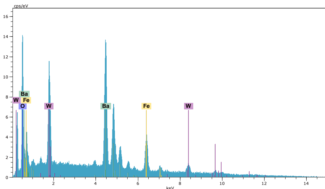
Slika 41. EDX spektar spoja Ba 3 Fe 2 WO 9 .
