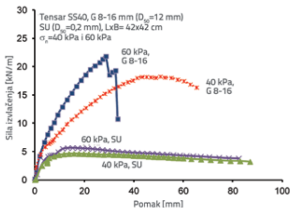
Slika 9. Razlike u sili izvlačenja za normalna naprezanja 40 i 60 kPa u šljunkovitoj pijesku i pijesku [3]
