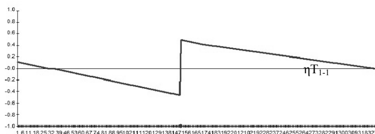
Slika 33 – Utjecajna linija riješena u Robotu za poprečnu silu u presjeku 1-1 na poduprtoj gredi
