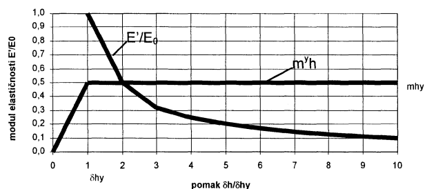
Slika 8. Idealizirani model nelinearnosti out-of-plane zidova
