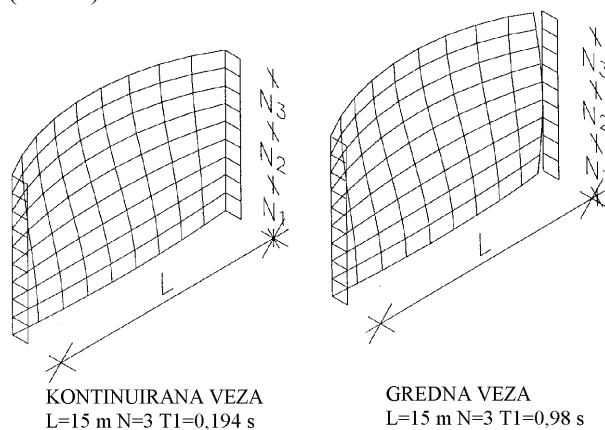
Slika 3. Usporedba odziva zida duljine L = 15\text{ m} i visine 9\text{ m} ( N = 3 ), za oba tipa uglovne veze
