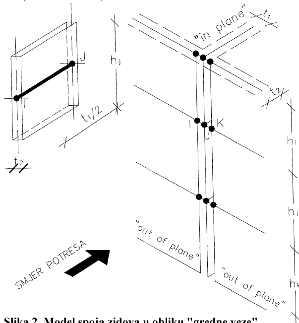
Slika 2. Model spoja zidova u obliku "gredne veze"
