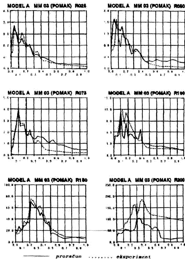
Slika 13. Usporedba eksperimentalnih i proračunanih spektara odziva modela bez krutih stropova za sve faze opterećenja
