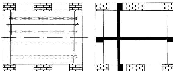
Slika 10. Pokus ZRMK. Tlocrti ispitanih modela
