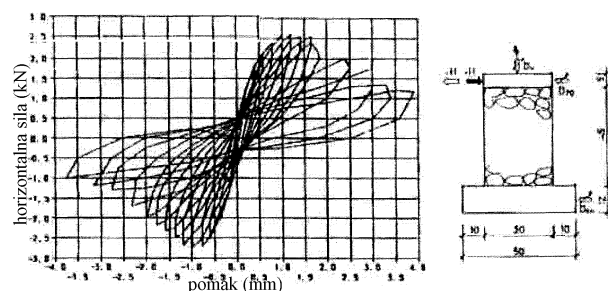
Slika 11. Pokus ZRMK. Prethodno ispitivanje zida
