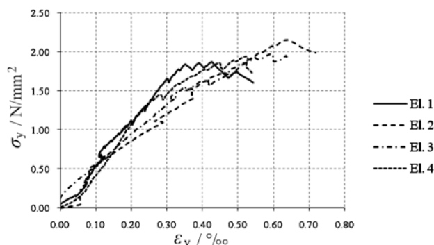
Figure 4 Relationship between normal strain and normal stress Slika 4. Odnos normalnog naprežanja i deformacije
