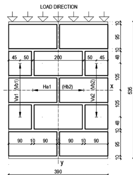
Figure 2 Front (back) side of the test specimen. Units are mm. Slika 2. Prednja (stražnja) ploha ispitnog uzorka. Jedinice su mm.
