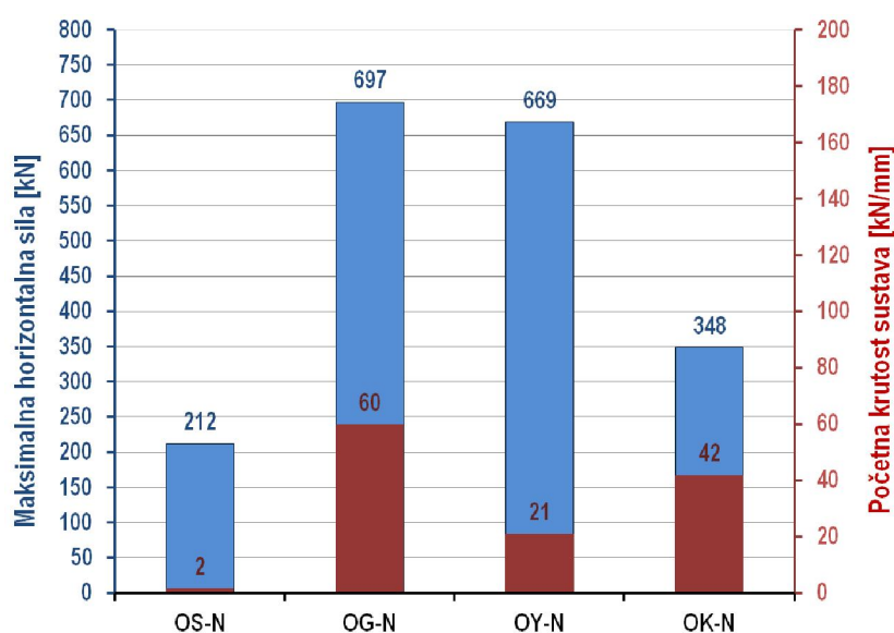
Slika 7.5 – Maksimalne dosegute horizontalne sile i početne krutosti sustava Oi-N
