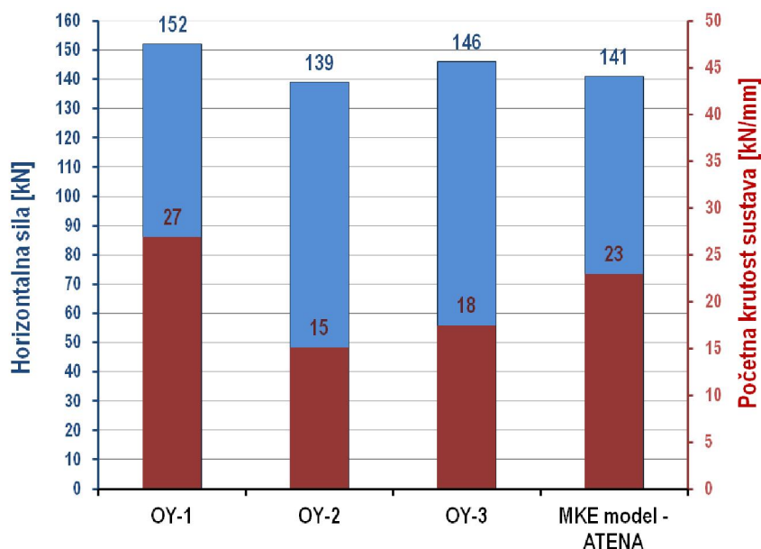
Slika 5.73 – Nosivost i krutost ispitivanih okvira OY-i i modela iz programskog paketa ATENA 2D
