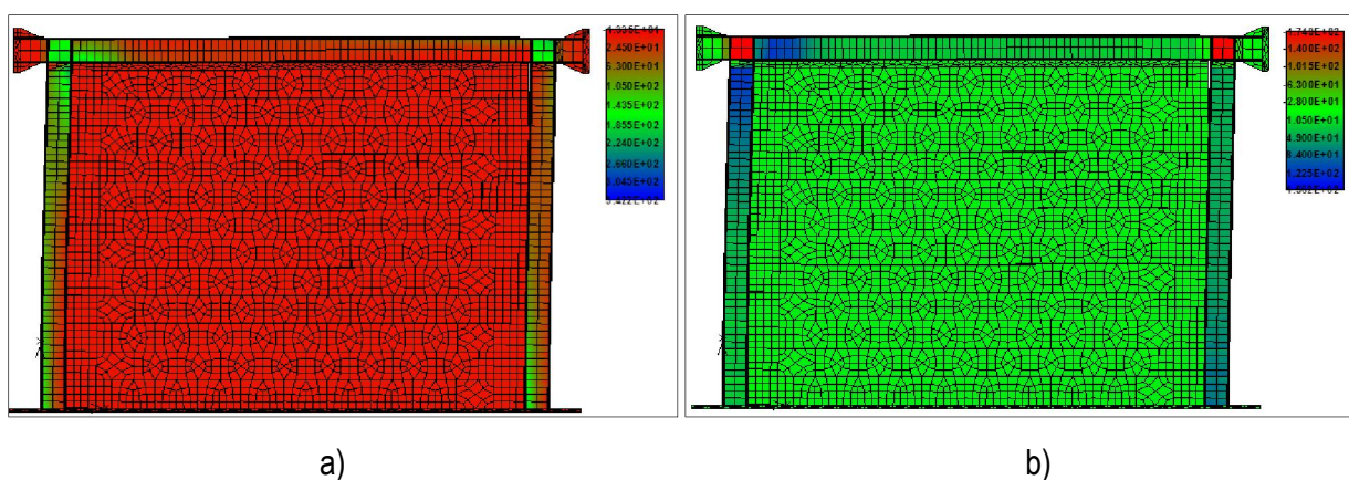
Slika 5.104 – Normalna (a) i posmična naprezanja (b) u čeličnom okviru pri međukatnom pomaku od 1,0 %
