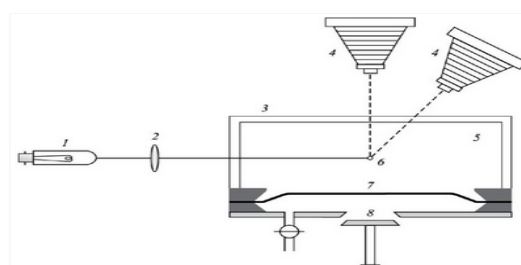
WILSONOVA KOMORA - 1. bjeskalica, 2. leća, 3. stakleno kućište, 4. fotoaparat, 5. prostor komore, 6. kondenzacijska jezgra, 7. pokretna membrana, 8. klip
