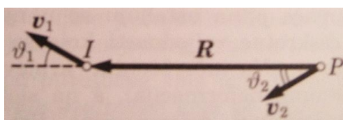
Slika 9: Vektorski prikaz relativnog gibanja [8]
