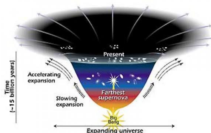
Slika 12: Brzina udaljavanja objekata u svemiru [16].
