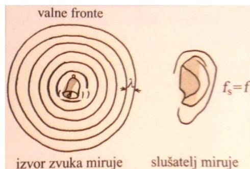
Slika 3: Valne fronte kada izvor i opažatelj miruju [10].
