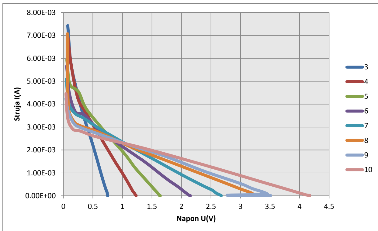
Slika 4.2.4. Dijagram ovisnosti napona o struji
