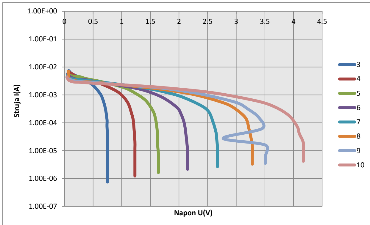
Slika 4.2.6: U-I karakteristika s log. podjelom na y-osi
