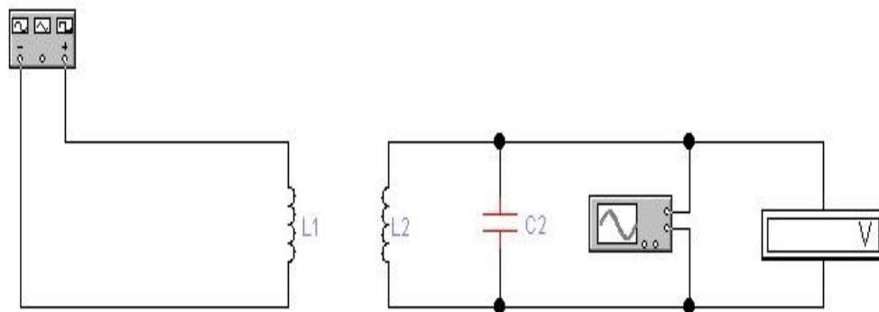
Slika 2.5. Električna shema
