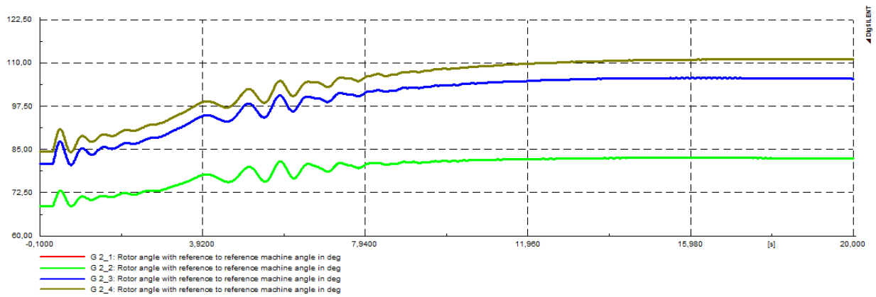
Sl. 7.53 Kratki spoj na vodu 10
