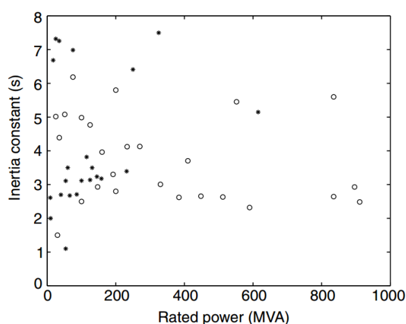
Slika 3.1 Inercijske konstante hidro jedinica (zvijezde) i parnih jedinica (krugovi) preko raspona nazivnih snaga prema različitim izvorima [1]
