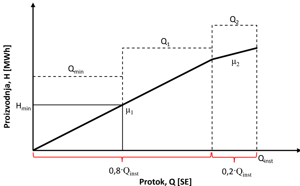
Sl. 4.1. Ulazno-izlazna karakteristika s označenim segmentima i pripadnim ekvivalentima proizvodnje
