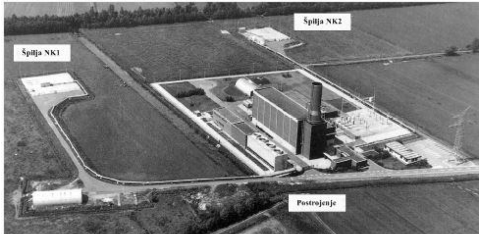
Slika 18. Huntorf postrojenje [3]
