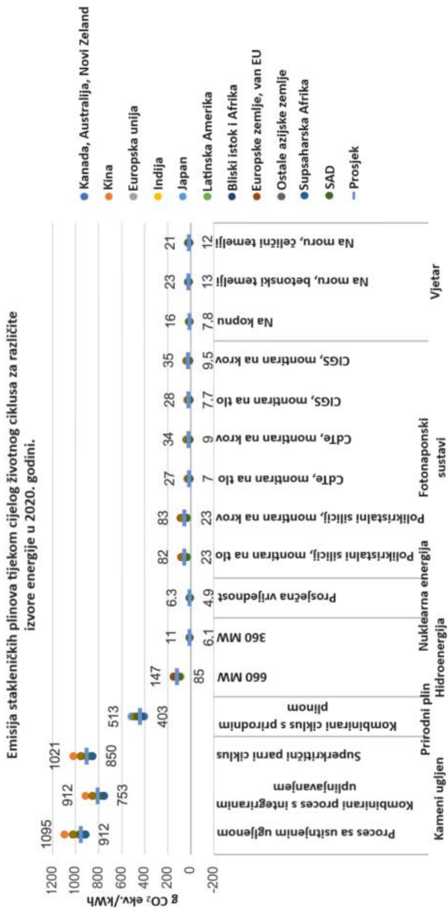
Slika 3.6. Emisija stakleničkih plinova tijekom cijelog životnog ciklusa za različite izvore energije u 2020. godini
