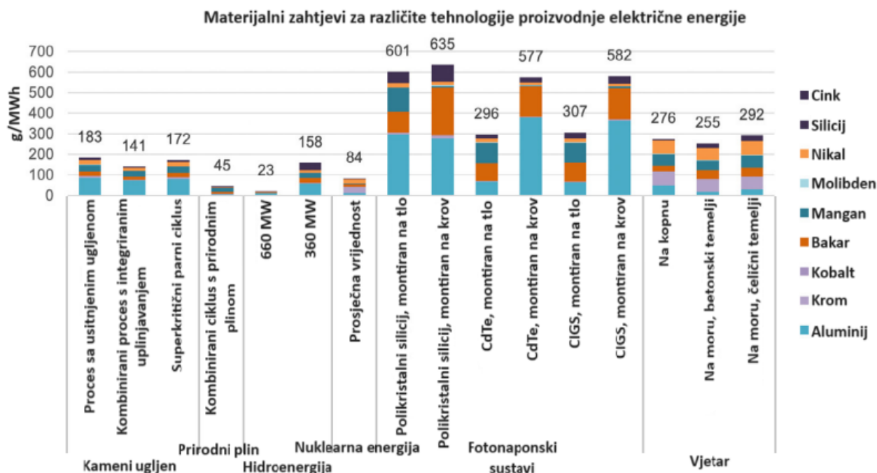
Slika 3.7. Materijalni zahtjevi za različite tehnologije proizvodnje električne energije [52]
