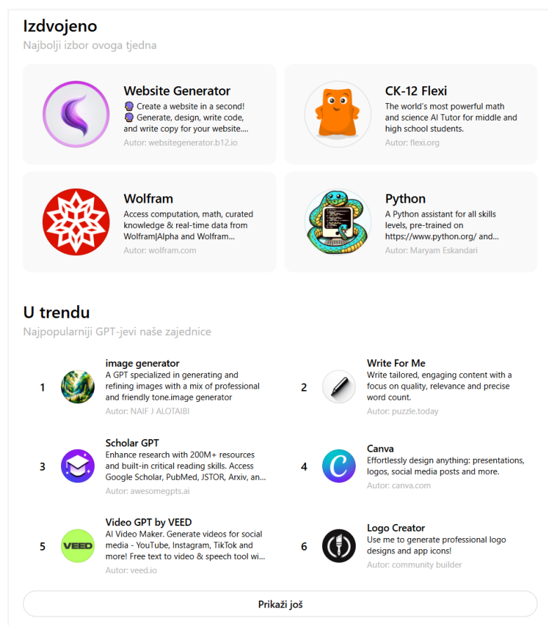
Slika 2.4. - Primjeri GPT-jeva
