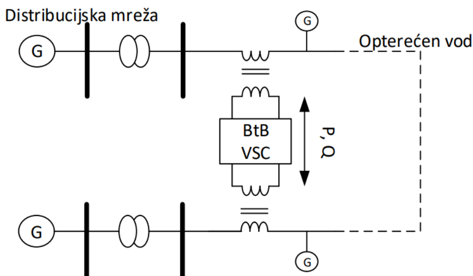
Slika 3.14. Uravnoteženje transformatora pomoću Btb veze [1]
