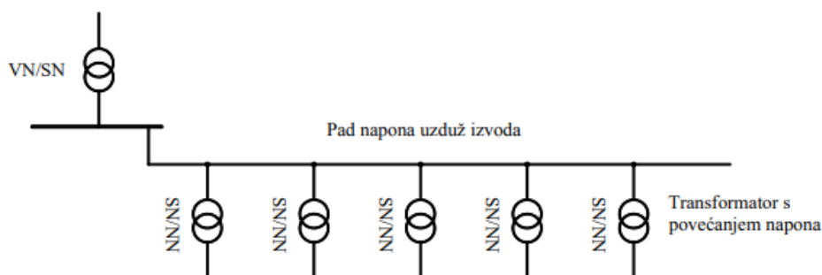
Slika 3.2. Osnovni princip kontrole napona u distribucijskoj mreži [1]
