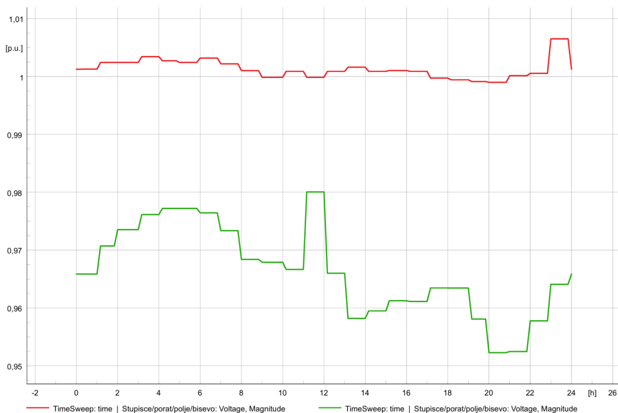
Slika 4.17. Utjecaj integracije male hidroelektrane na napon na električki najudaljenijoj sabirnici
