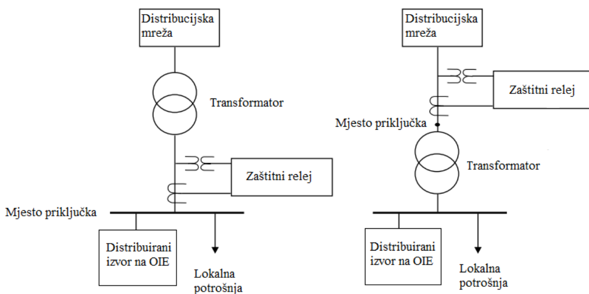
Slika 2.3. Dvije vrste priključka distribuiranog izvora [1]
