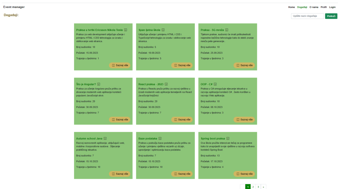
Slika 5.5. Komponenta EventsComponent
