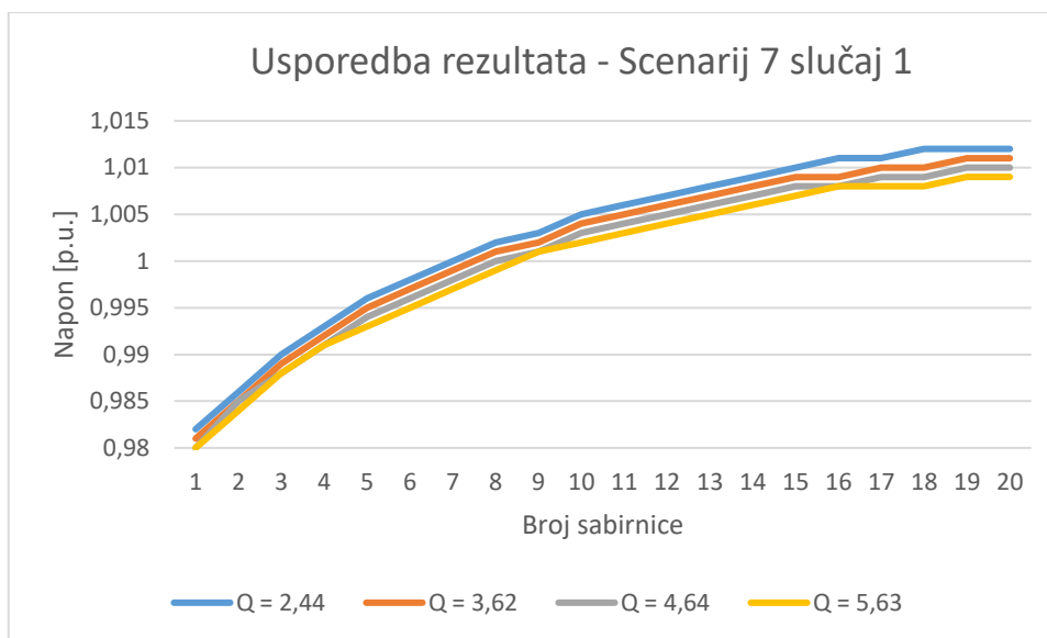
Slika 4.78. Usporedba rezultata – Scenarij 7 slučaj 1
