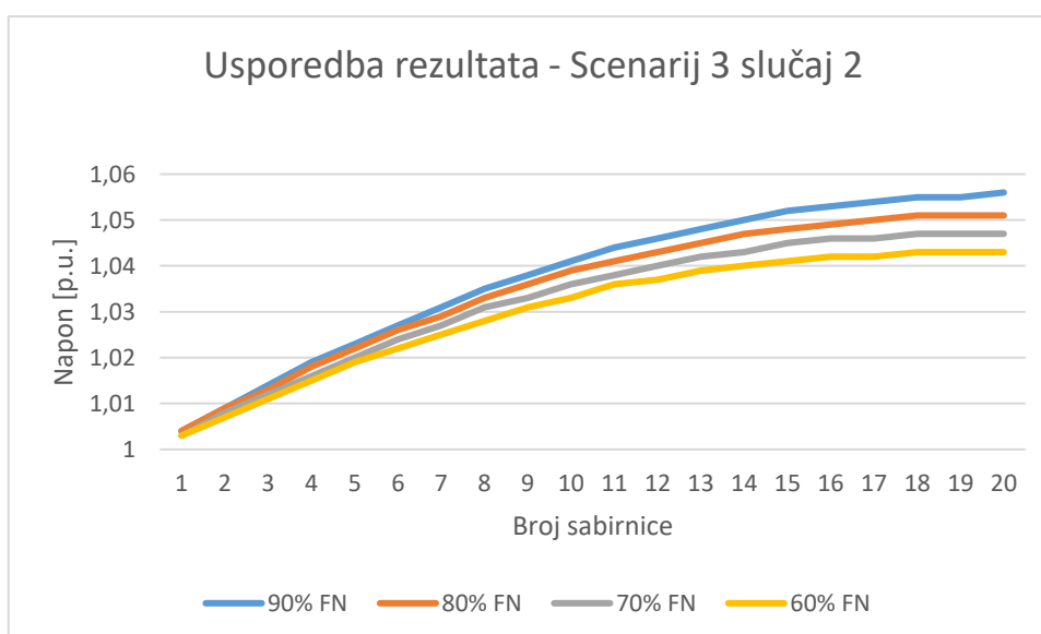
Slika 4.54. Usporedba rezultata – Scenarij 3 slučaj 2
