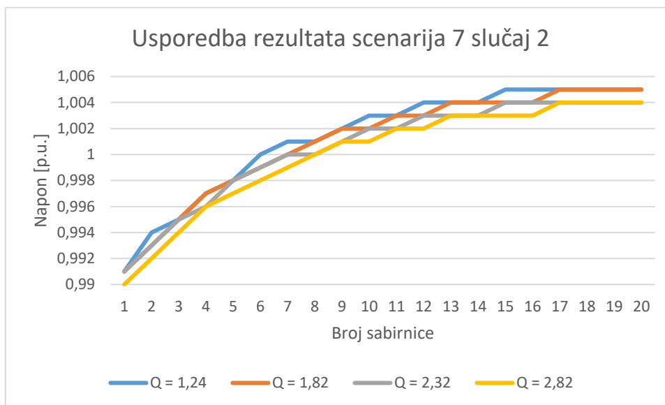
Slika 4.94. Usporedba rezultata – Scenarij 7 slučaj 2
