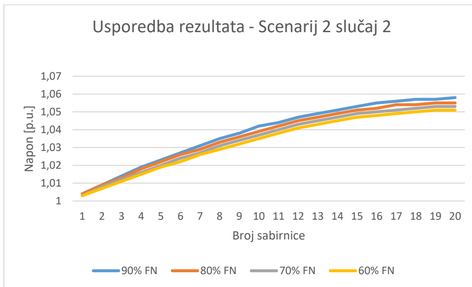
Slika 4.48. Usporedba rezultata – Scenarij 2 slučaj 2
