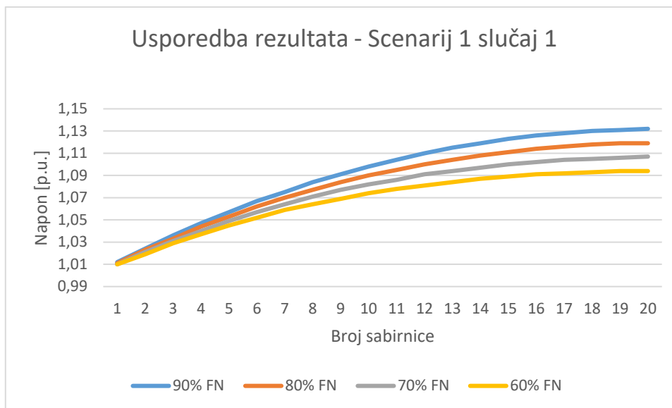
Slika 4.12. Usporedba rezultata – Scenarij 1 slučaj 1
