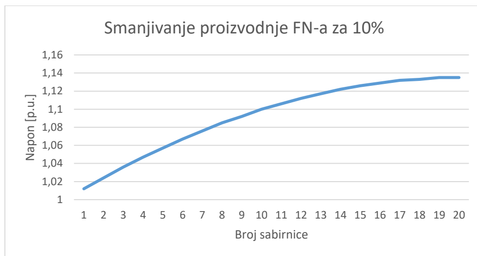
Slika 4.26. Napon na sabirnicama pri 90 % proizvodnje FN-a na svakoj drugoj sabirnici svakog izvoda (maksimalna proizvodnja FN-a)
