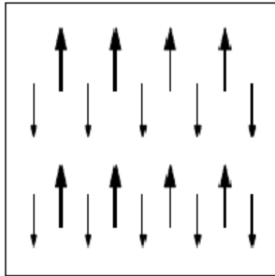
Slika 2.8. Prikaz magnetskih momenata unutar domene ferimagnetskog materijala [12]
