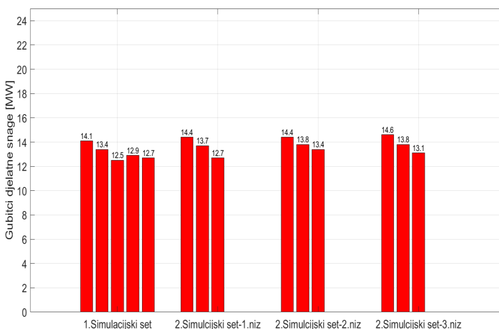
Slika 6.10. Prikaz ukupnih gubitaka djelatne snage za sve simulacijske slučajeve.
