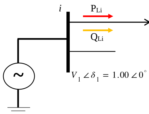
Slika 3.4. Referentni čvor.
