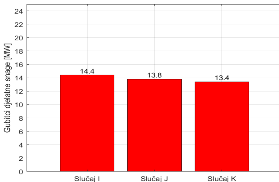
Slika 6.6. Prikaz ukupnih gubitaka djelatne snage za drugi niz 2. seta simulacijskih slučajeva. Grafički prikaz rezultata simulacija za posljednji niz simulacijskih slučajeva dan je na slikama 6.7. i 6.8. Na slici 6.7. se kao i u prethodnom razmatranju primjećuje veće odstupanje napona po slučajevima kroz koje se mijenja samo pozicija referentne sabirnice. Može se vidjeti kako su
