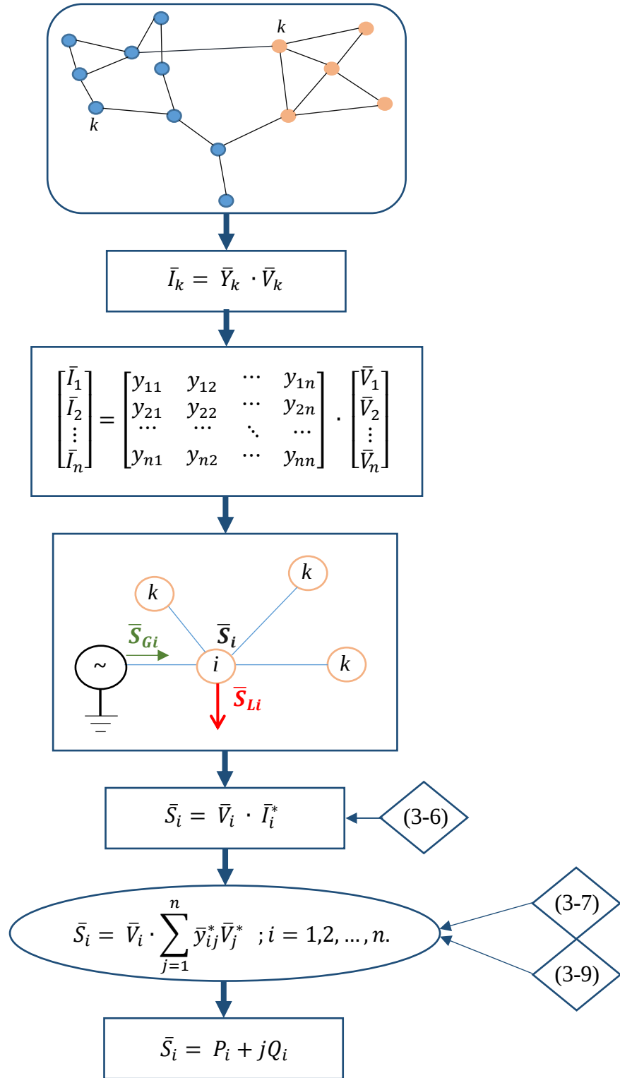
Slika 3.1. Dijagram toka formulacije jednađbi za tokove snaga.
