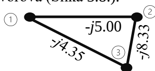
Slika 3.8. Admitancije mreže.
