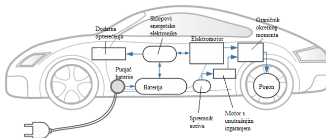
Slika 3. 9. Konfiguracija paralelnog pogona[20]
