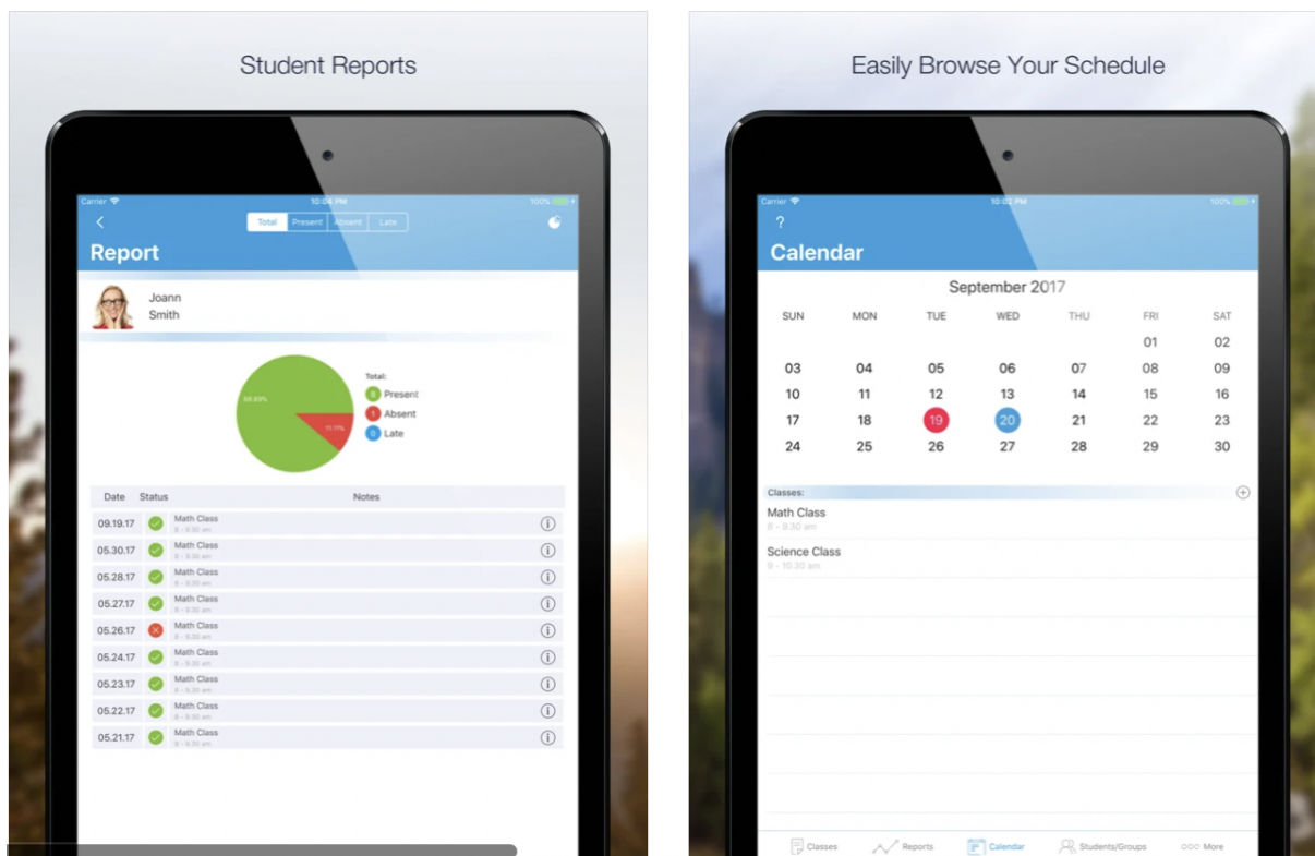
Slika 2.3. Alora aplikacija
