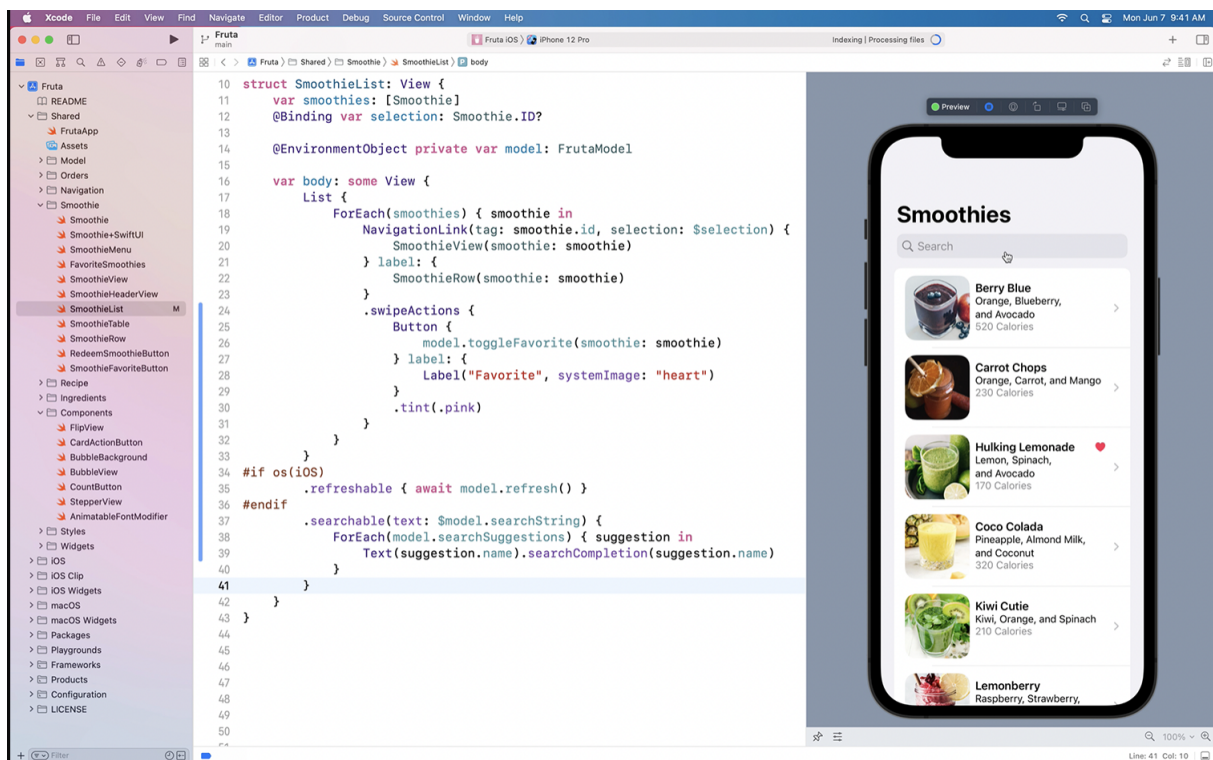
Slika 3.2. SwiftUI
