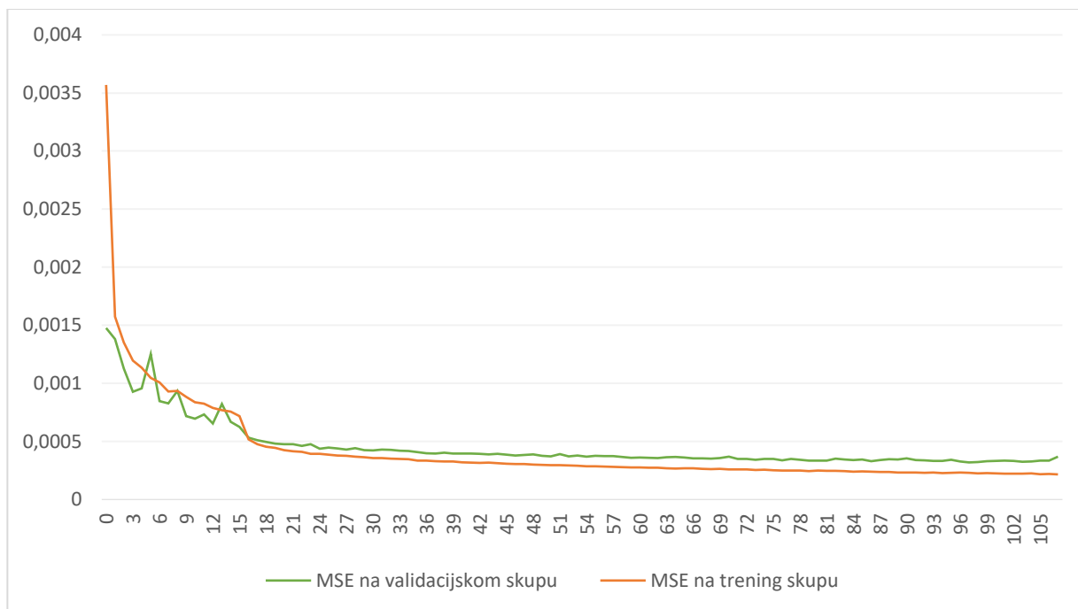
Sl. 3.15. Graf promjene kriterijske funkcije (MSE) kroz epohe treninga mreže
