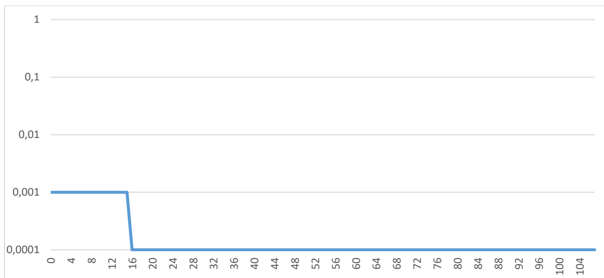
Sl. 3.16. Graf promjene stope učenja kroz epohe treninga mreže
