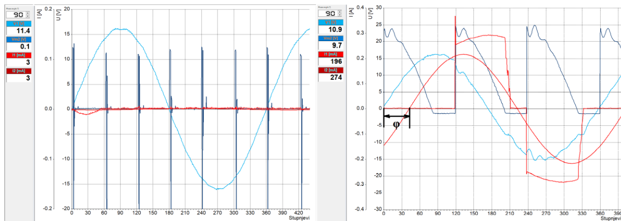
Sl. 5.3. Valni oblici karakterističnih napona i struja punoupravljevog spoja (lijevo) i poluupravljevog spoja (desno) za kut 90^\circ el.
