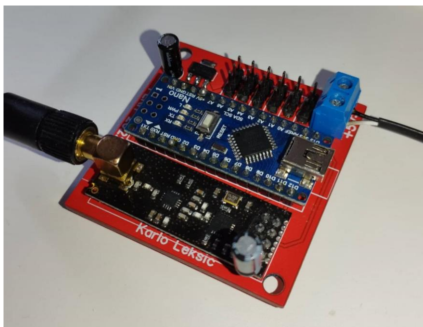
Sl. 3.11. PCB za prijemnik.
