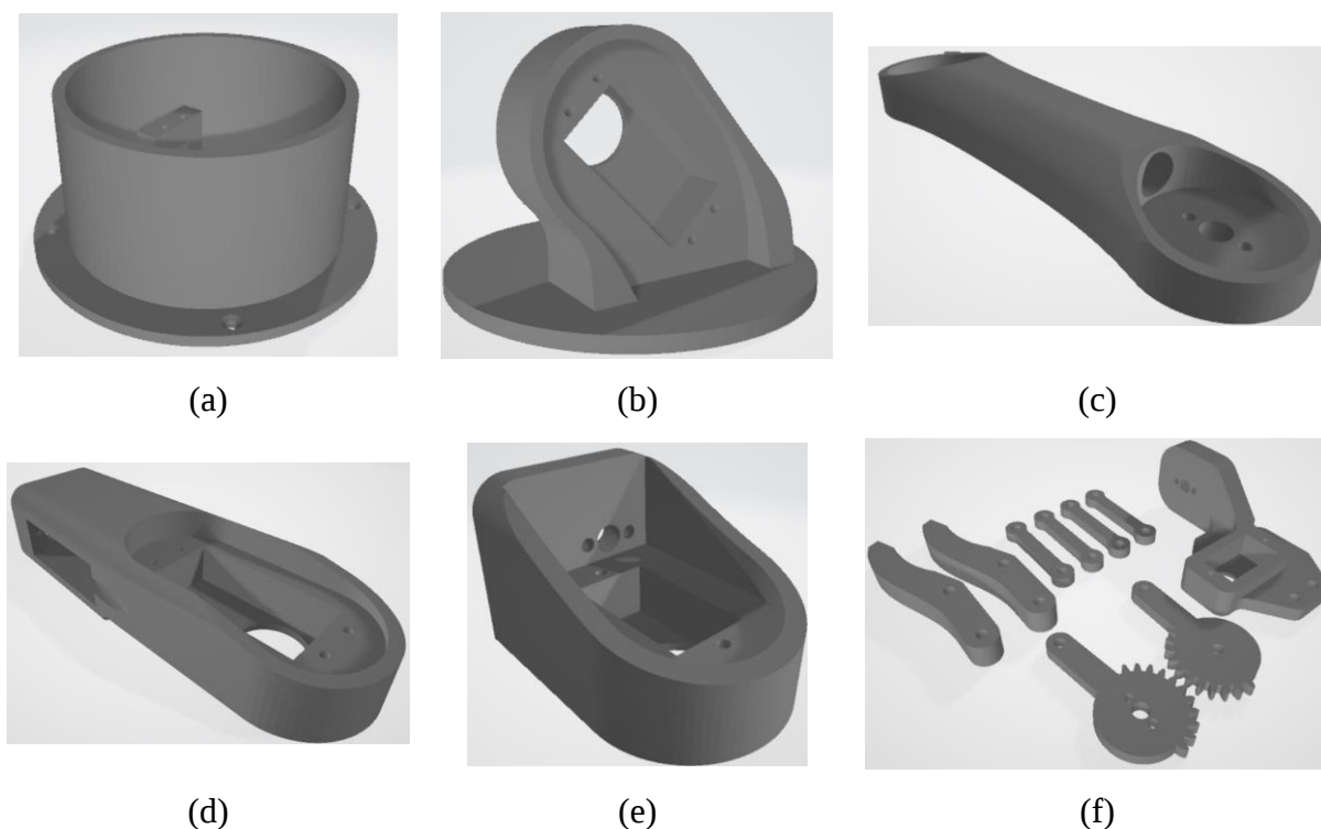
Sl. 3.1. Glavni dijelovi 3D modela robotske ruke, postolje (a), poveznica 1 (b), poveznica 2 (c), poveznica 3 (d), poveznica 4 (e) i hvataljka (f).
